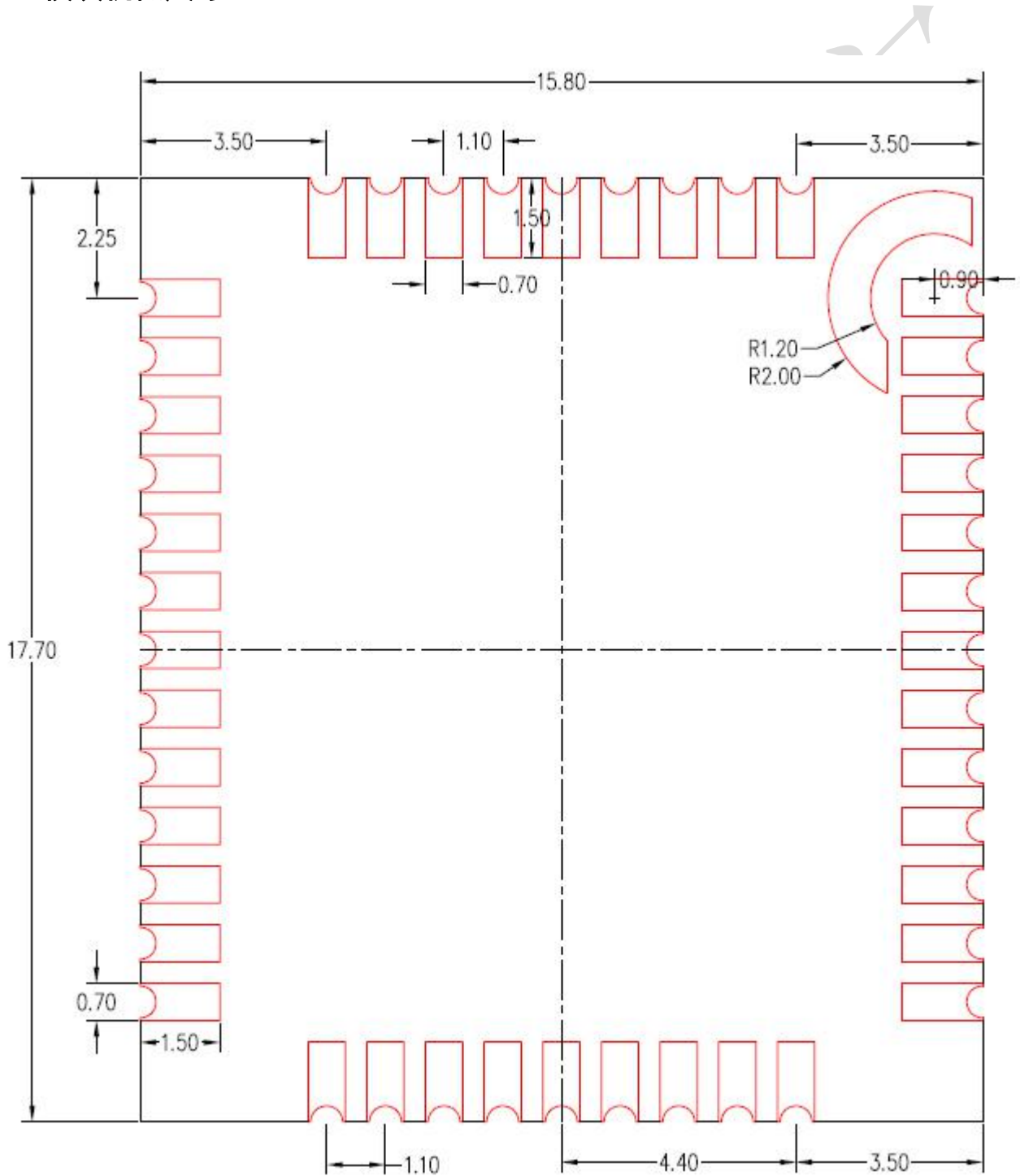
图表 28: Air208M 正视图 (单位: 毫米)
